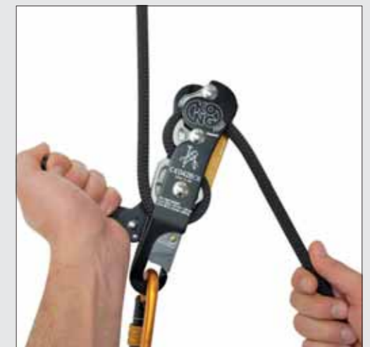
Locking by pulling Bloccaggio a freno
